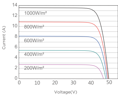
Current-Voltage Curve(SAS540M- 144H )
