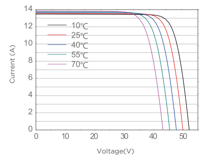
Current-Voltage Curve(SAS540M- 144H )
