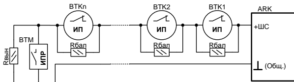
Рисунок Б4. Схема пожарного ШС с несколькими тепловыми извещателями ВТК (типа ИП105).
