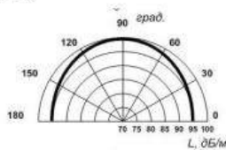
Рисунок 1 – Диаграмма направленности оповещателя
